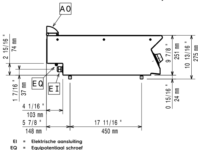
Boven aanzicht
